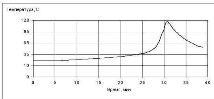
Стандартная экзотермическая кривая для MA422 при 23°C (10 грамм) 5
